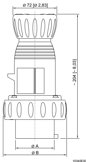
8571/12 Wtyczka SolConeX
