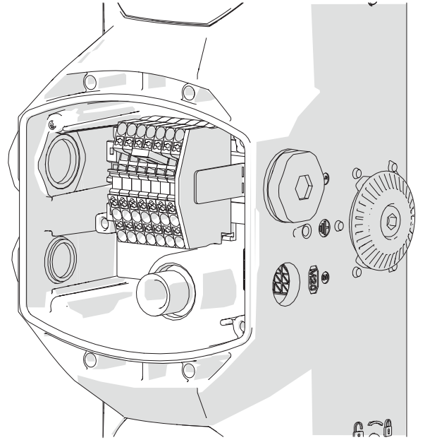
Chambre de connexion Ex e
