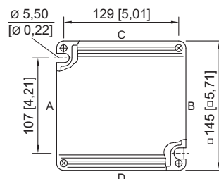
8118/.3. Gehäuse Gr. 3
