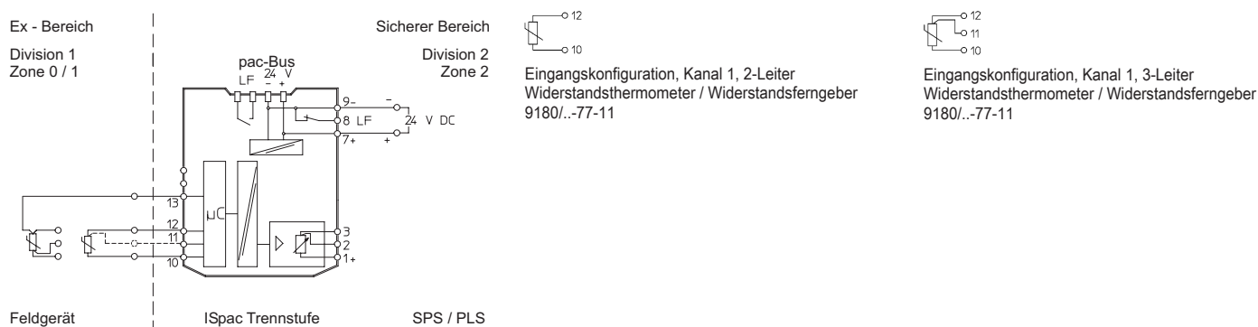
Anschlussplan 9180/1.-77-11
