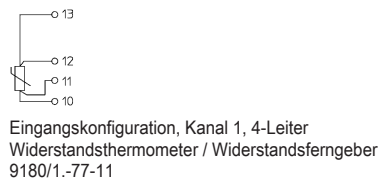
Anschlussplan 9180/1.-77-11
