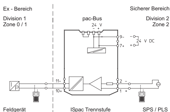
Anschlussplan 9165/16-11-10
