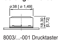
8003/...-001 Drucktaster
