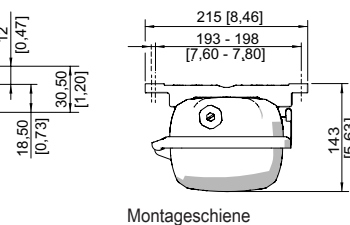
Montagebügel
