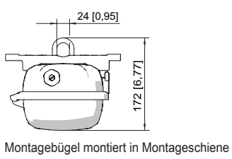
Montageschiene
