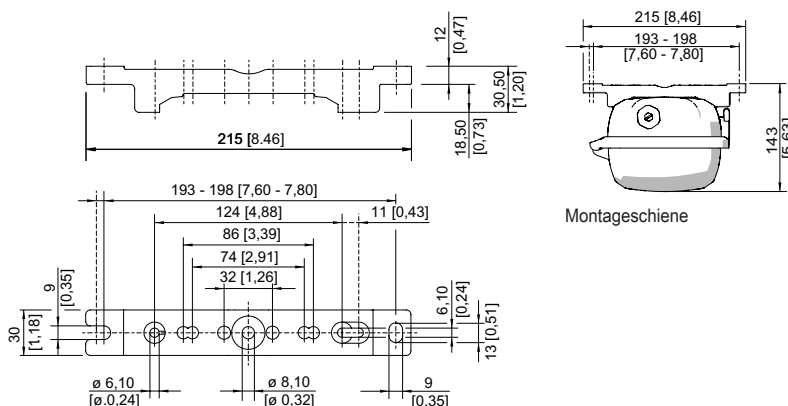
Montageschiene
