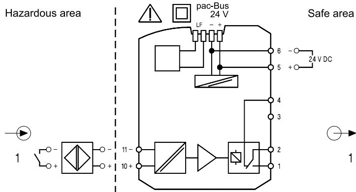
Anschlussbild 9270/11-16-14
