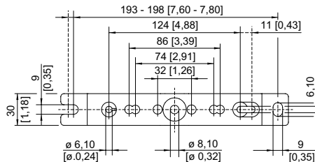
Montageschiene
