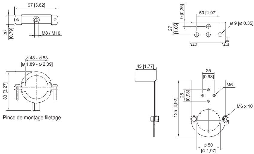
Pince de montage surface
