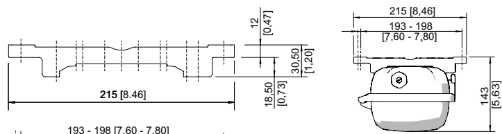
Raíl de montaje DIN
