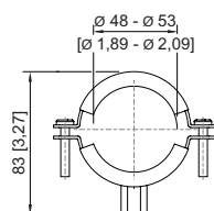
Abrazadera de montaje para rosca
