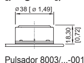
Pulsador 8003/...-001
