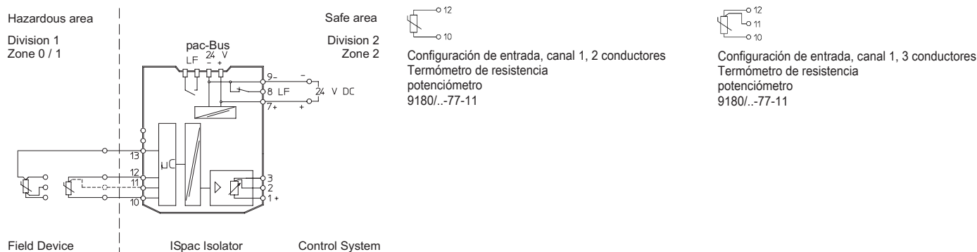
Diagrama de conexión 9180/1.-77-11
